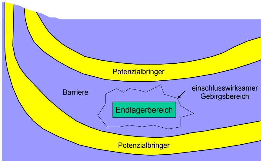
Abbildung 5-3: Schematische Darstellung von Potenzialgebieten und Endlagerbereich 35
