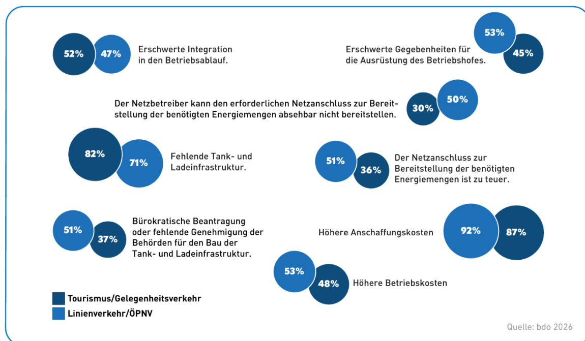
Abb. 5: bdo-Sonderabfrage – Umstiegshürden
