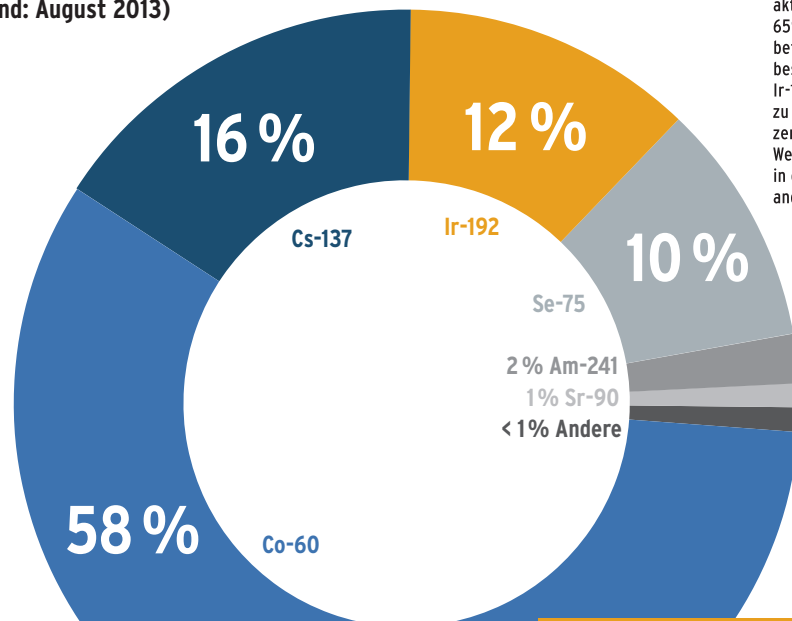
Anteil der jeweiligen Nuklide in hochradioaktiven Strahlenquellen in Deutschland (Stand: August 2013)
