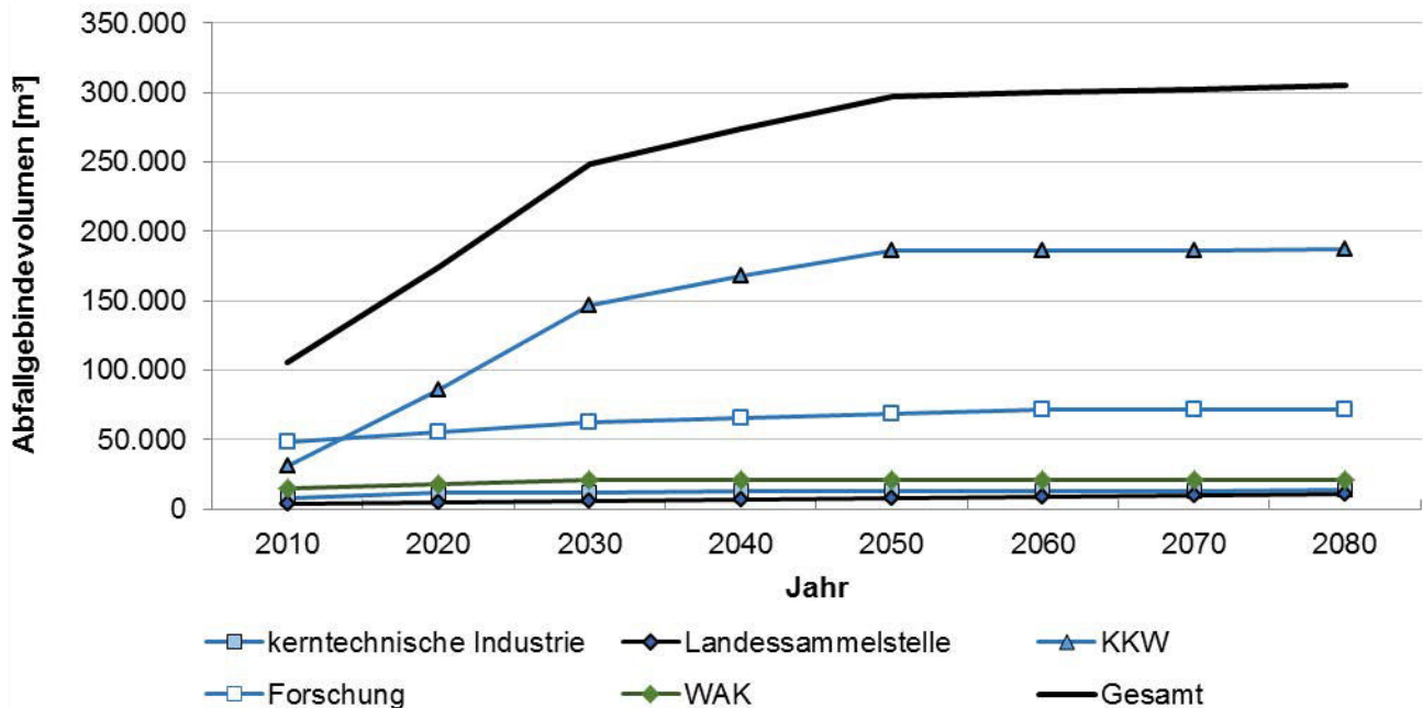
Abbildung D-15: Zeitlicher Verlauf des kumulierten Anfalls radioaktiver Abfälle mit vernachlässigbarer Wärmeentwicklung als Abfallgebindevolumen bis zum Jahr 2080
